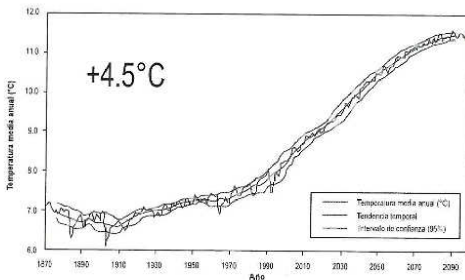
Gráfico N° 4: Variación de la temperatura a nivel mundial (Período 1870 – 2090)
